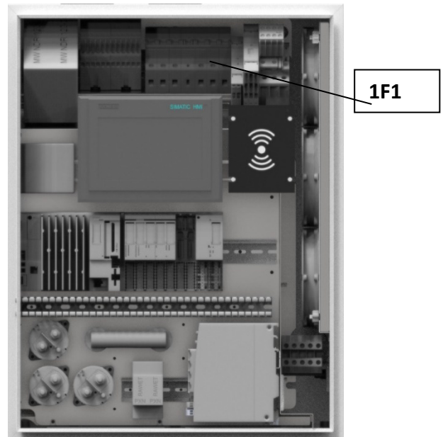
Abb 10: 1F1 Leitungsschutzschalter
