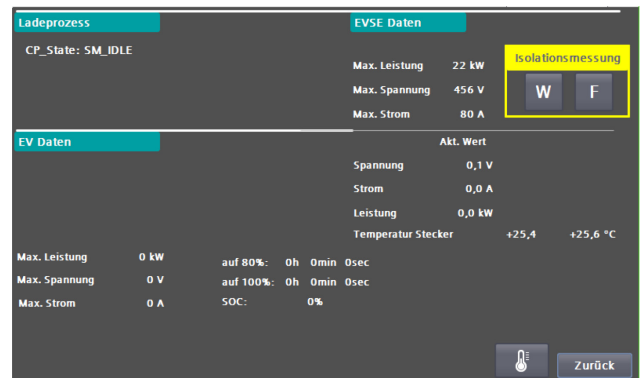
Abb 46: Ladung CCS/CHAdeMO
