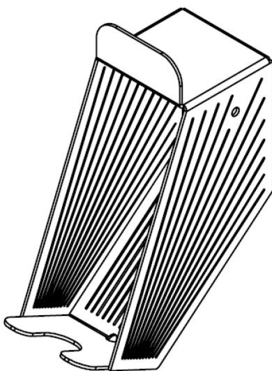
Abb 8: Ladesteckerhalterung CCS/CHAdeMO
