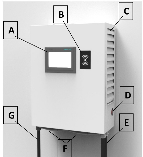
Abb 1: Ansicht Kostad DC-Wallbox
