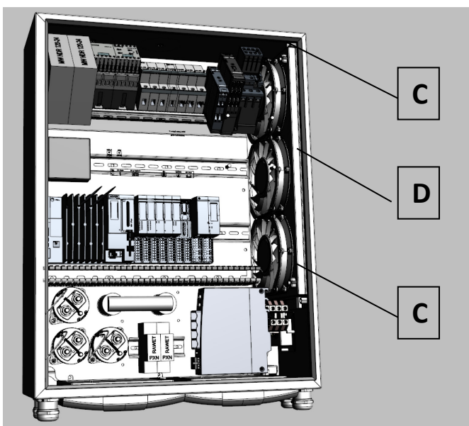
Abb 51: Innenansicht
