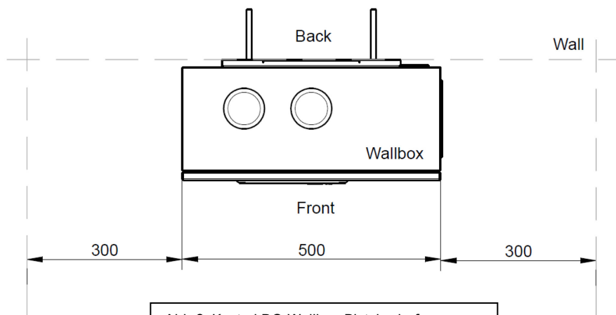
Abb 3: Kostad DC-Wallbox Platzbedarf
